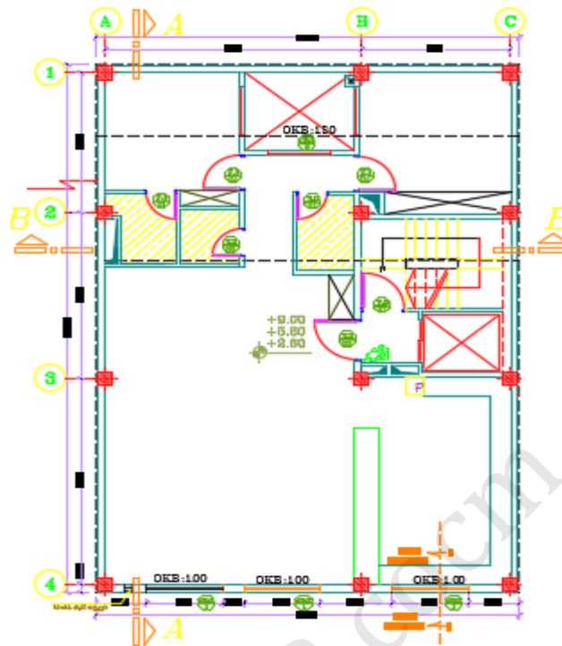
پلان تایپ طبقات
