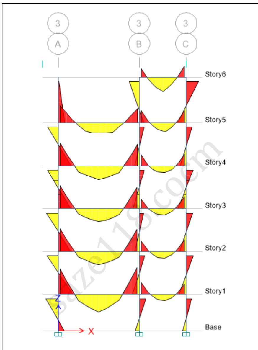
نمایش دیاگرام لنگر داخلی المانها حول محور ۳-۳
