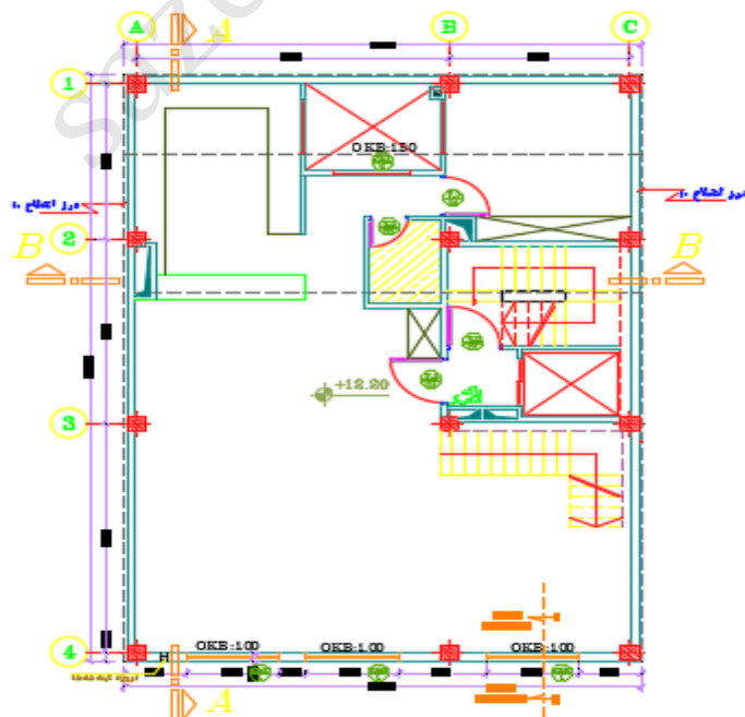
پلان طبقه ۴
